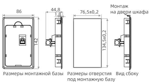
Установочные размеры HD-KMB
