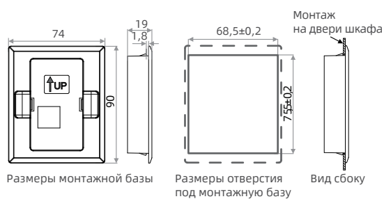
Установочные размеры HD-KMB-S
